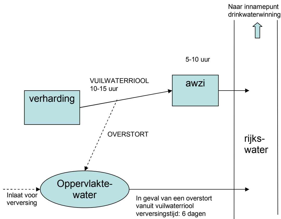
Figuur 2. Schematisch overzicht van de routes waarlangs regenwater uit het stedelijke gebied wordt afgevoerd bij een gemengd rioelstelsel, met geschatte verblijftijden voor elke onderdeel van de route
